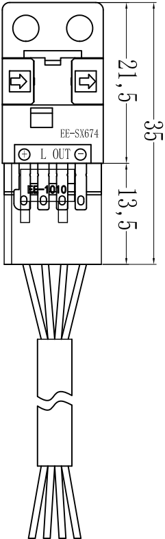
EE-1010/EE-SX674嵌合示意图
