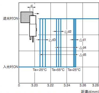
重复检测位置特性 EE-SX47□/67□
