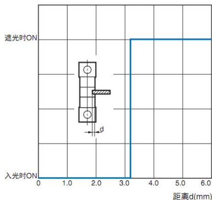
检测位置特性 EE-SX47□/67□
